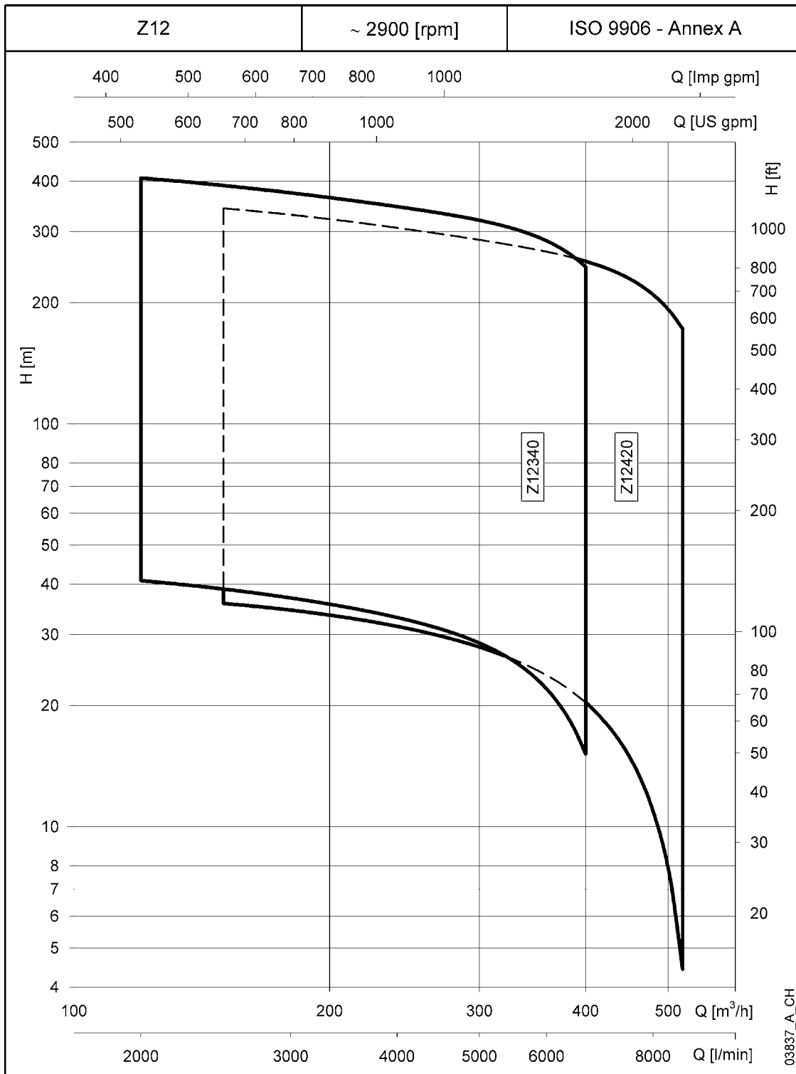
Capaciteitengrafiek Z12 serie bij 50 Hz, 2-polig
