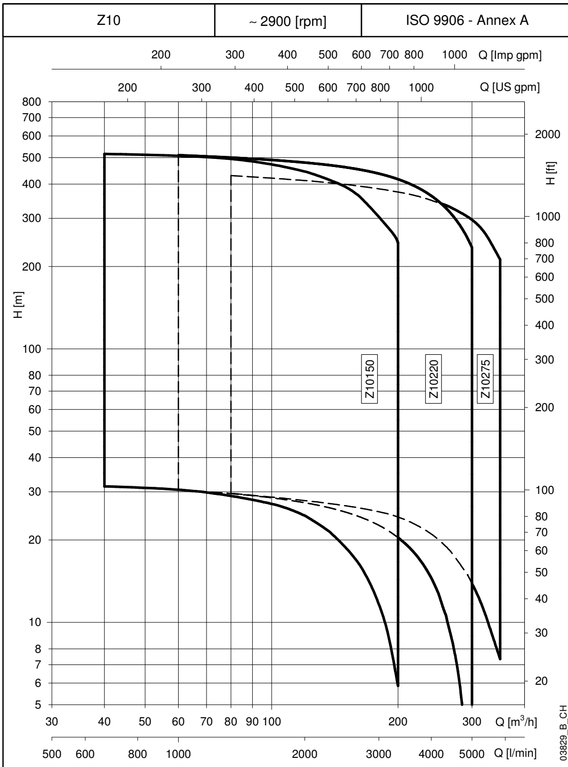
Capaciteitengrafiek Z10 serie bij 50 Hz, 2-polig
