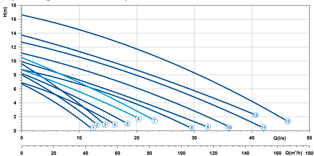
Capaciteitengrafiek V serie 50 HZ rpm 1450
