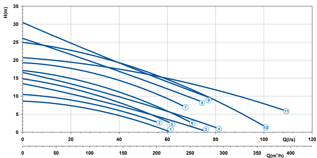
Capaciteitengrafiek serie V 50 HZ R.P.M. 1450 - 950
