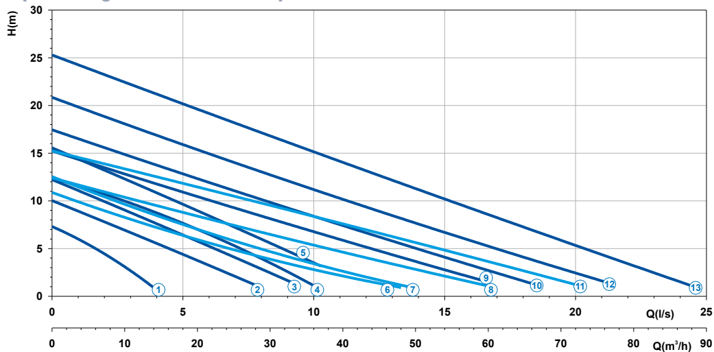
Capaciteitengrafiek V serie 50 HZ rpm 2850
