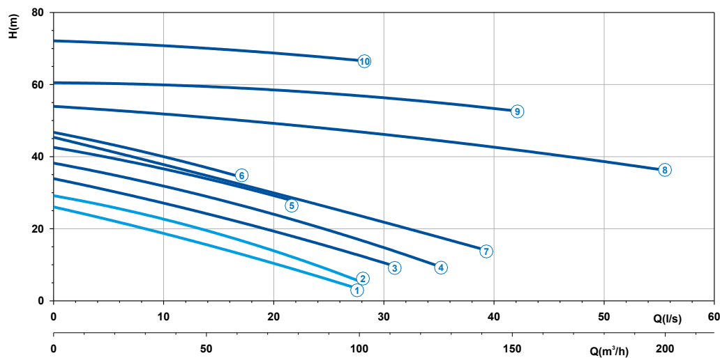
Capaciteitengrafiek V serie 50 HZ rpm 2850
