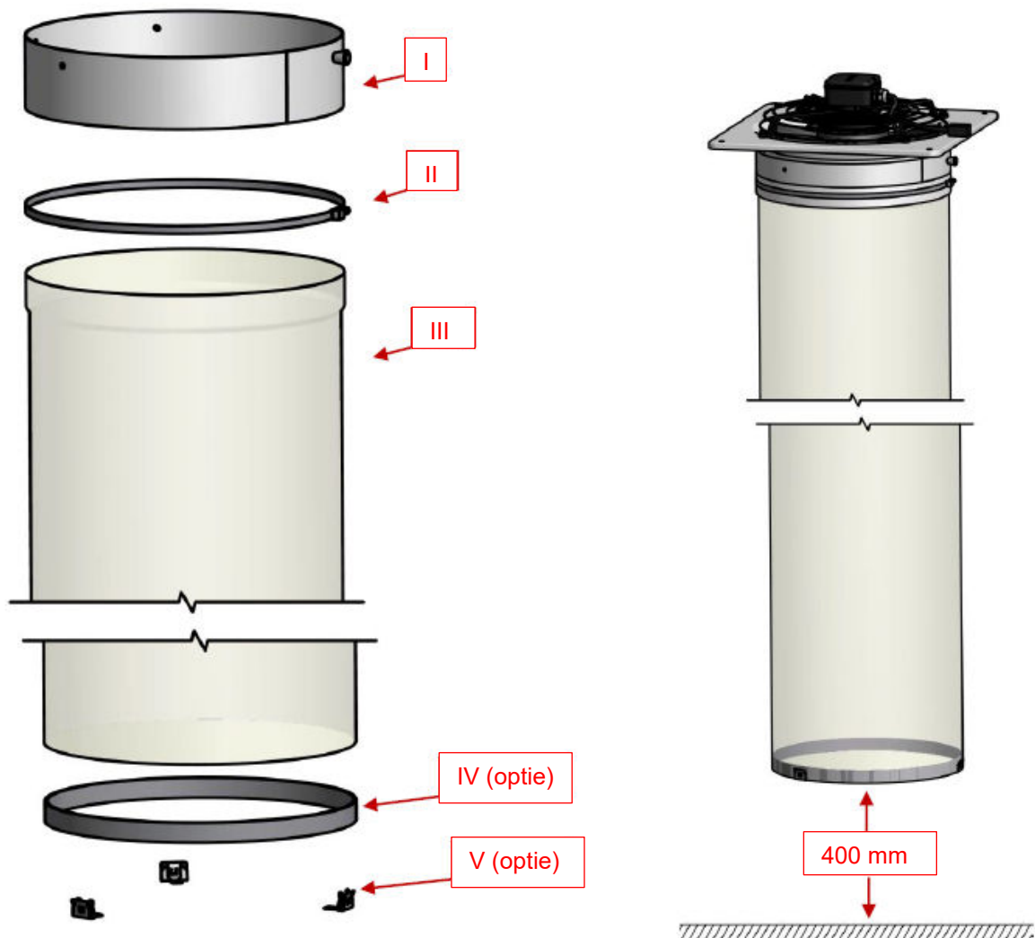
Afbeelding 9: Opbouw slurf
