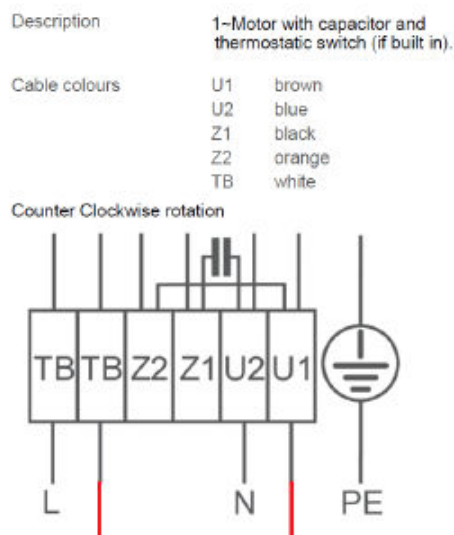
Figuur 10: Aansluitschema
