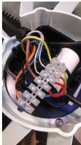
Figuur 11: Aansluiten thermisch contact
