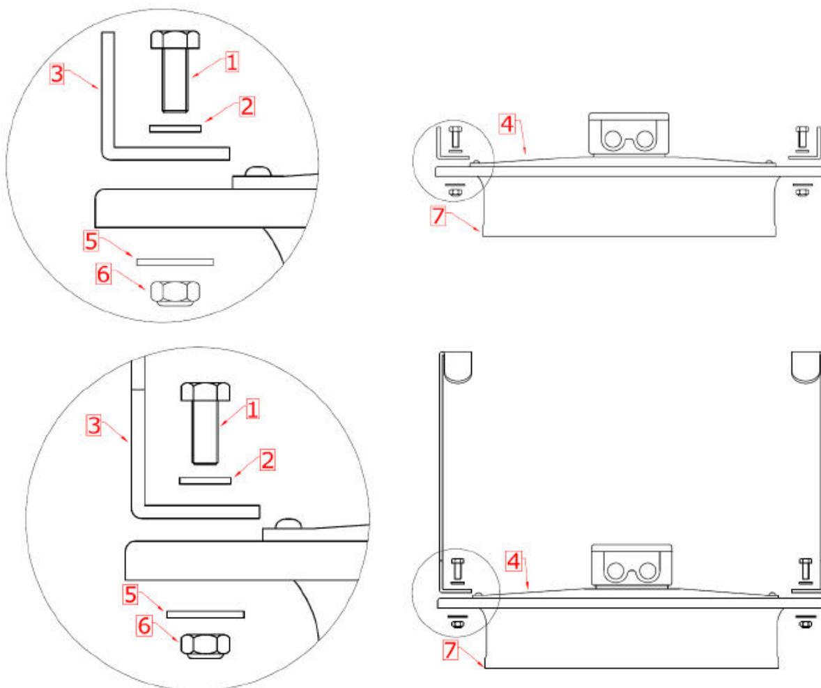
Afbeelding 6: Montage van de hoekprofielen of verlaagde beugel
