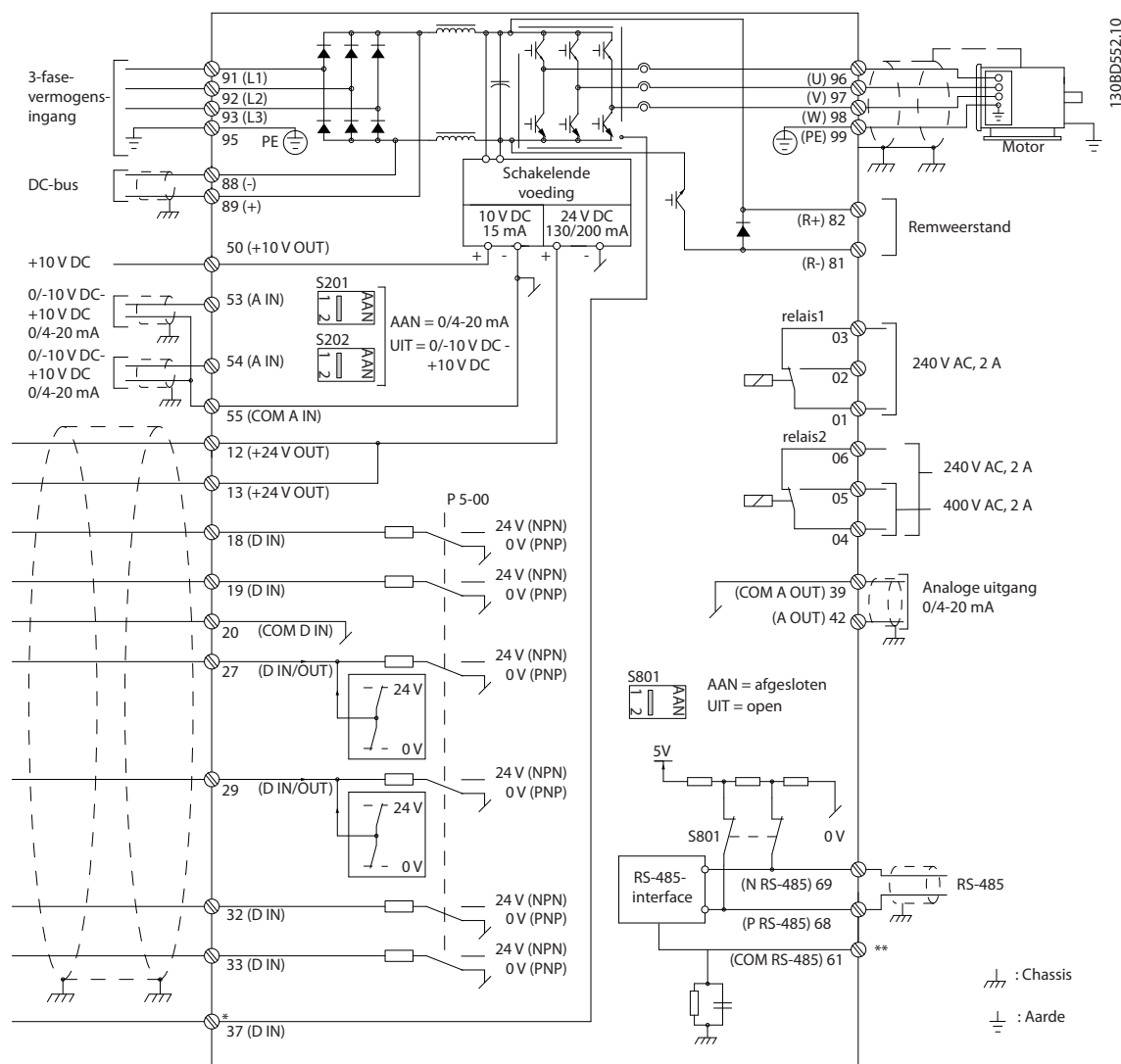
Afbeelding 4.1 Eenvoudig bedradingsschema
