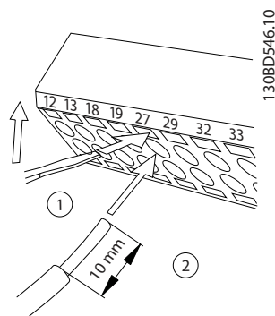
Afbeelding 4.12 Stuurkabels aansluiten
