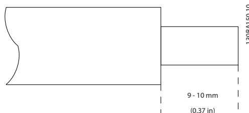
Afbeelding 6.50 Kabel strippen
