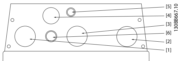
Afbeelding 6.28 B1 – IP 55
