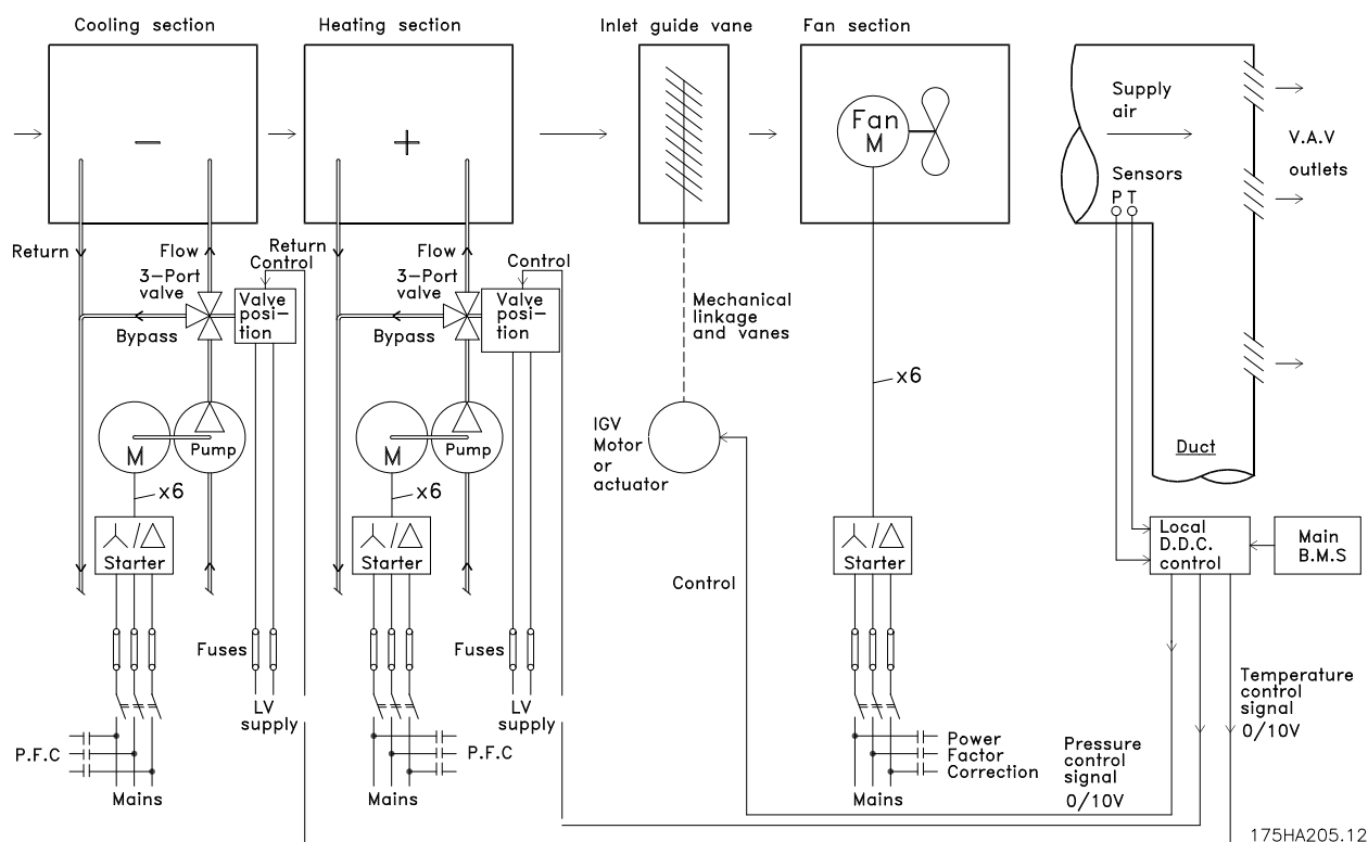
Afbeelding 2.15 Traditioneel ventilatorsysteem
