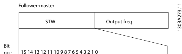
Afbeelding 8.16 Statuswoord
