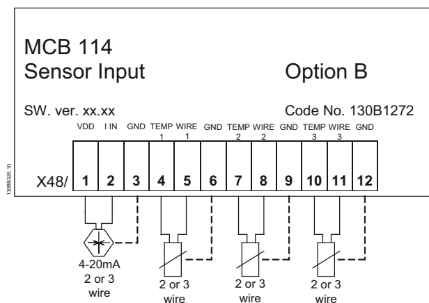
Afbeelding 3.15 Elektrische bedrading
