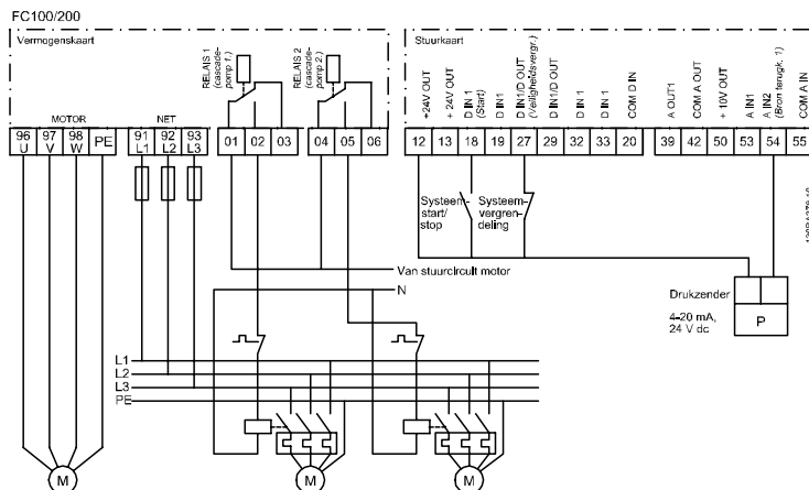
Afbeelding 7.11 Bedradingsschema cascaderelelaar
