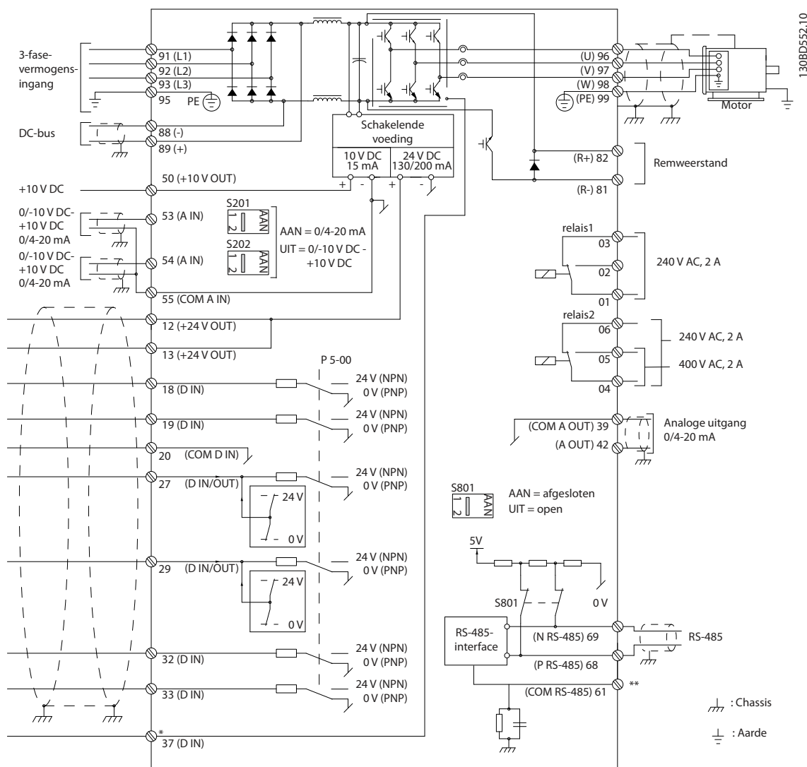
Afbeelding 6.55 Eenvoudig bedradingsschema
