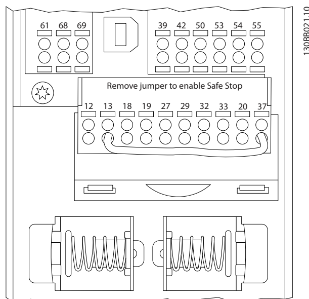
Afbeelding 8.2 Stuurkaartklemmen
