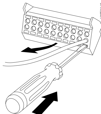
Afbeelding 6.52 Kabel insteken
