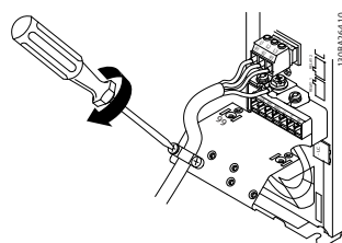
Afbeelding 6.5 De steunbeugel vastzetten
