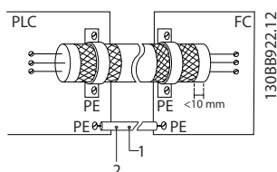
Afbeelding 6.65 Stuurkabel met vereffeningskabel
