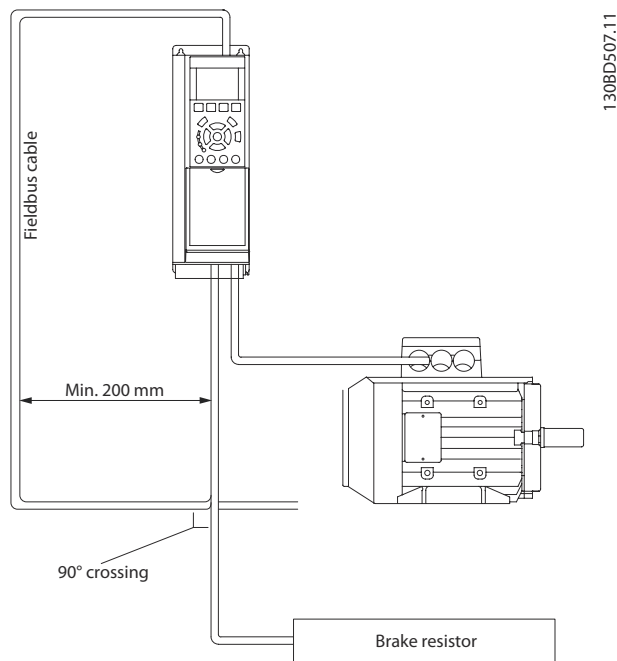
Afbeelding 8.4 Bekabeling
