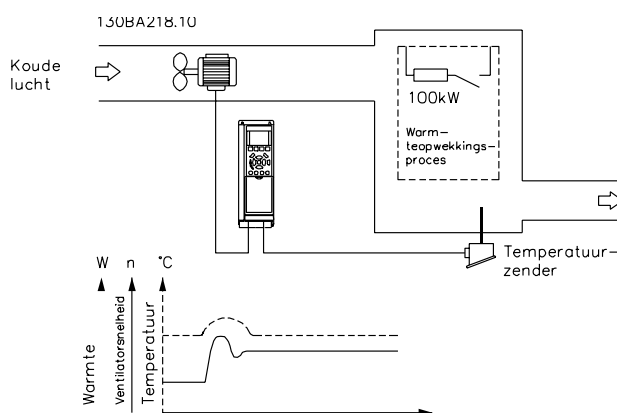
Afbeelding 2.30 Terugkoppelingsregeling voor een ventilatiesysteem
