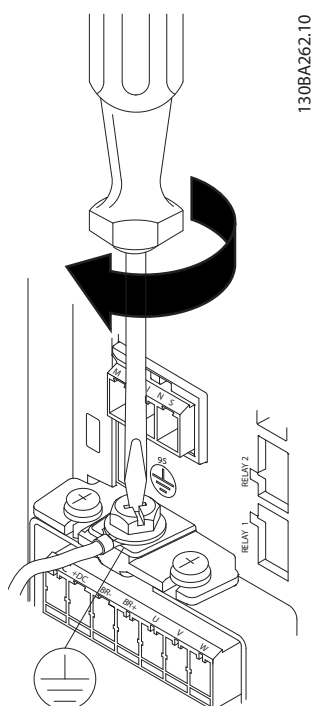
Afbeelding 6.3 De aardkabel vastzetten
