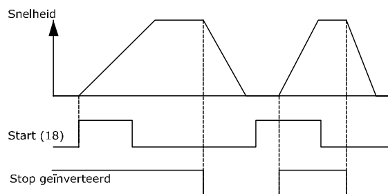
Afbeelding 6.54 Eenvoudige bedrading
