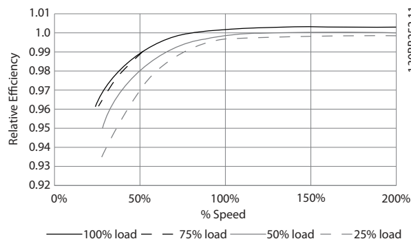
Afbeelding 9.2 Typische rendementscurves
