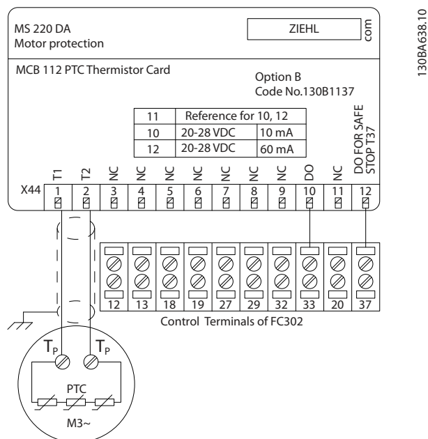
Afbeelding 3.13 MCB 112 installeren
