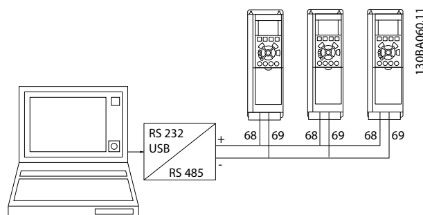
Afbeelding 8.1 Parallelle aansluitingen
