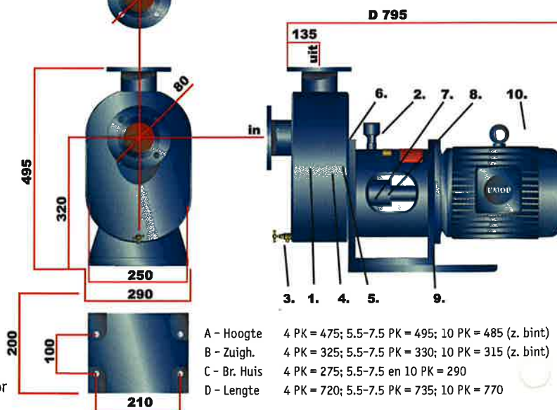
Maatschets en onderdelenlijst Goan type DA • 4-, 5.5-, 7.5- en 10 PK
